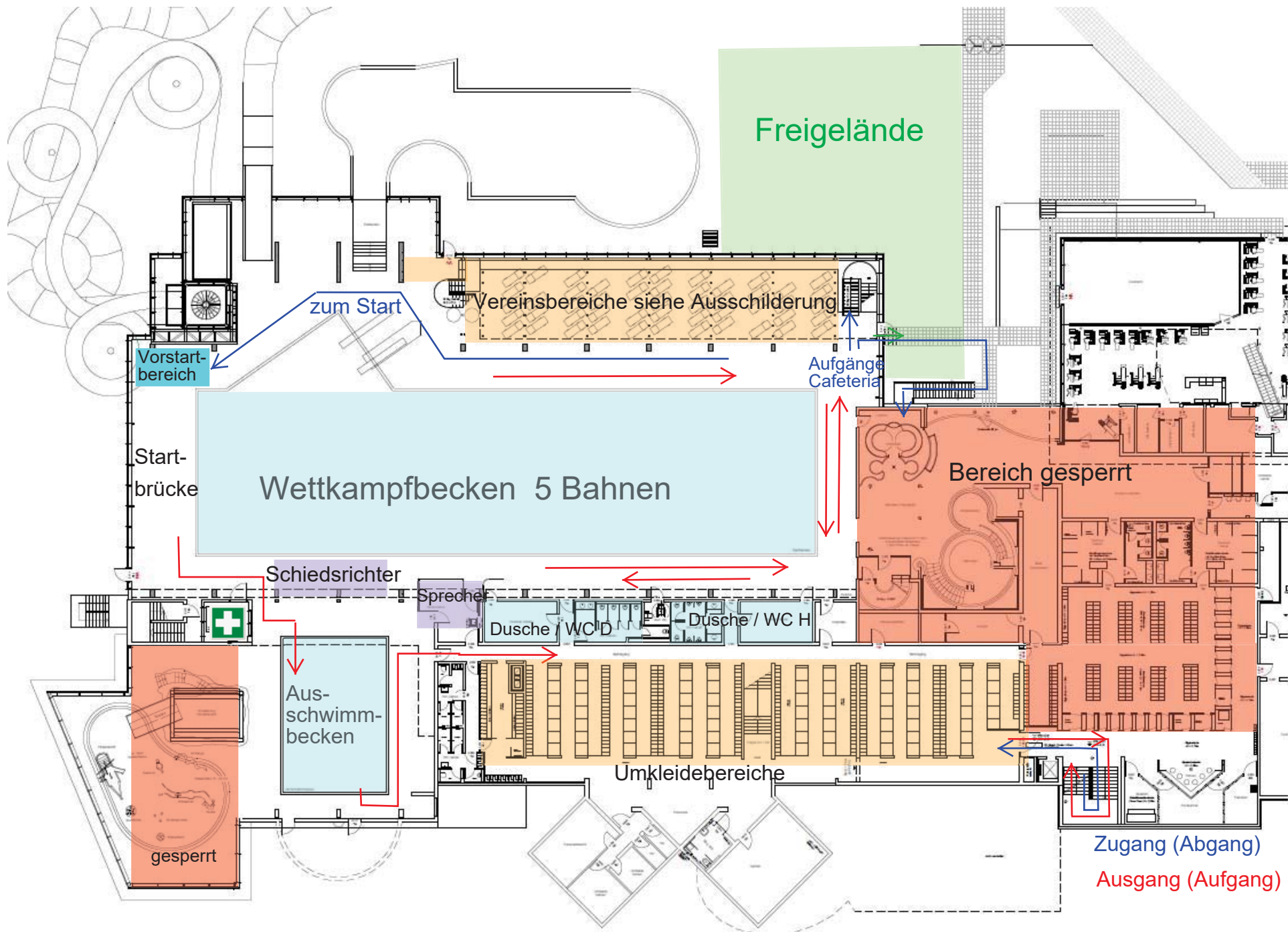
Plan Erdgeschoss, Schwimmhalle
